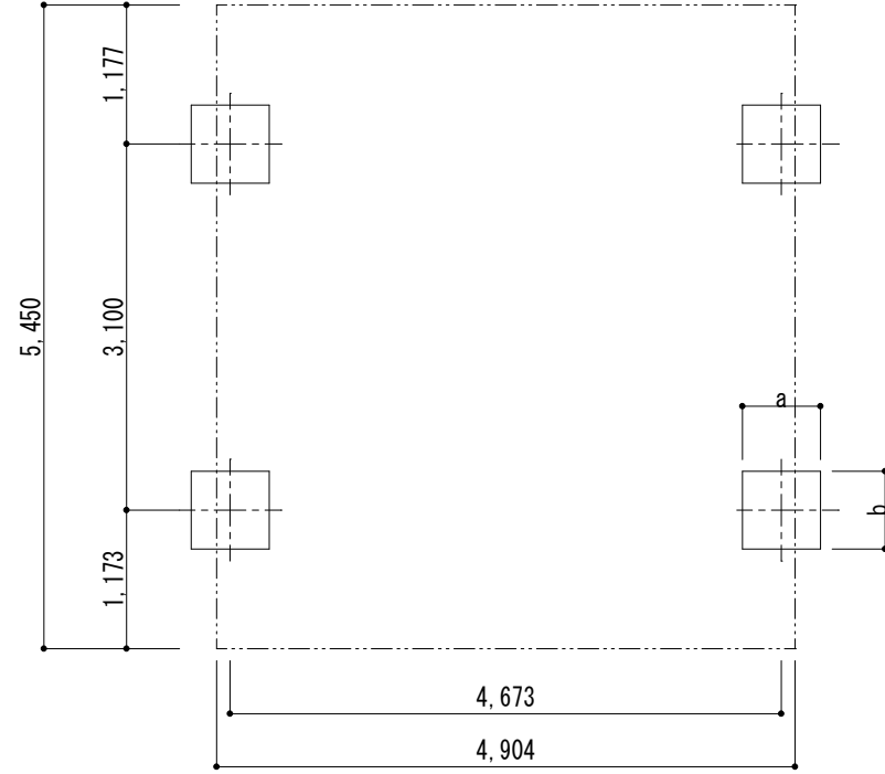
■ 基礎配置図
